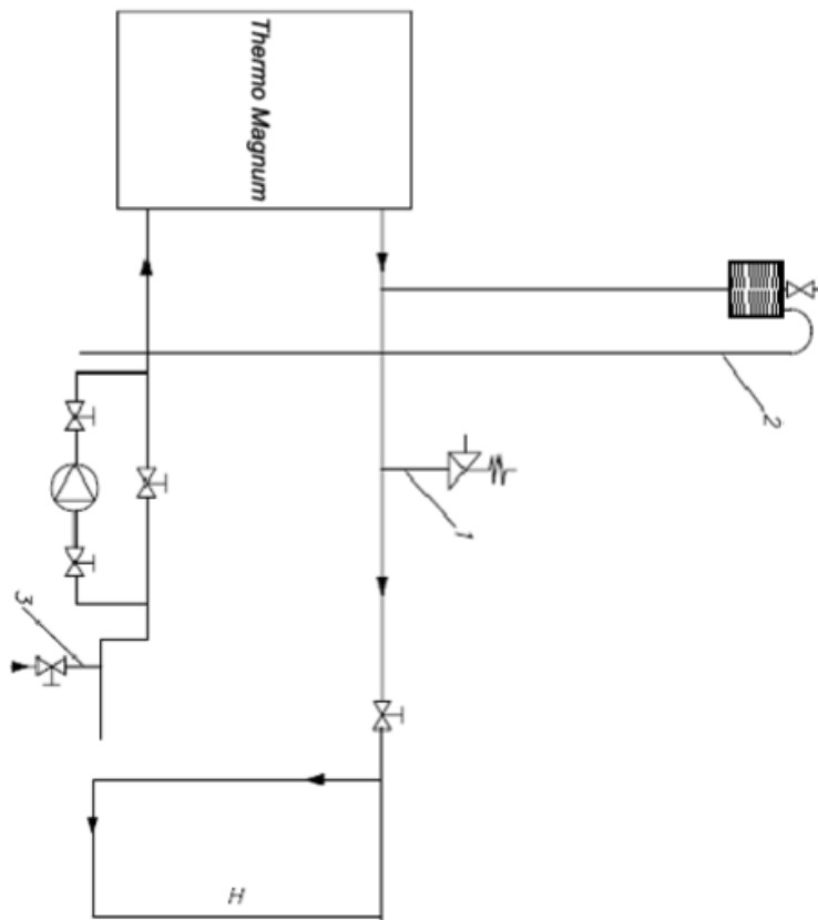
Schéma du système fermé de chauffage central (l'image 5)
