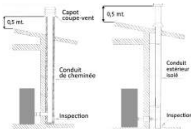
Fig. 2: raccord au conduit de cheminée
